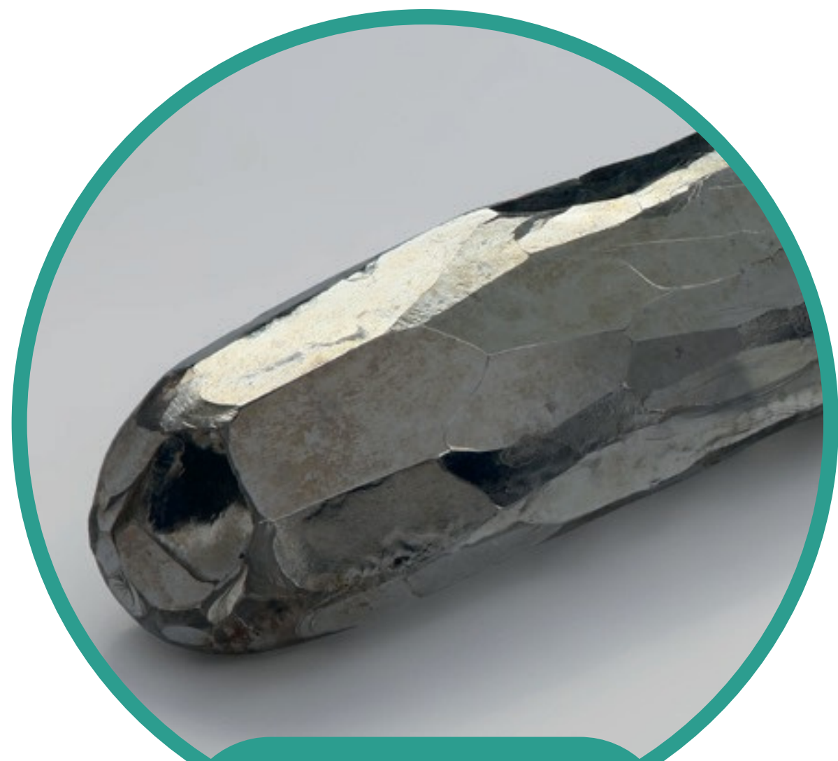
Cádmio
